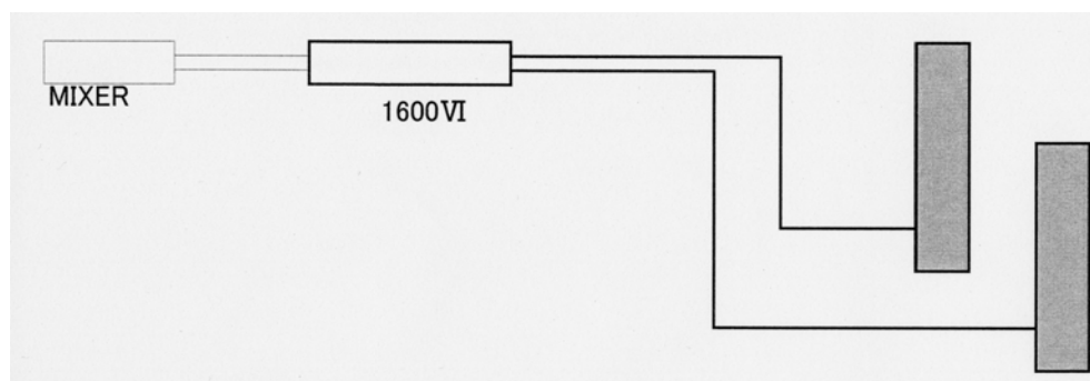
Line Array System LA1612×2本 三脚スタンド SS-5 II × 2本使用
