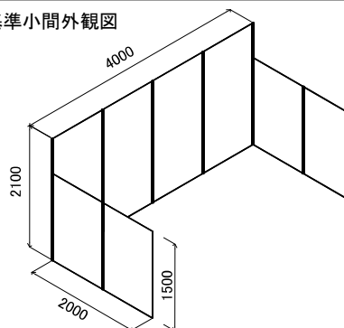
基礎パネル設営図
